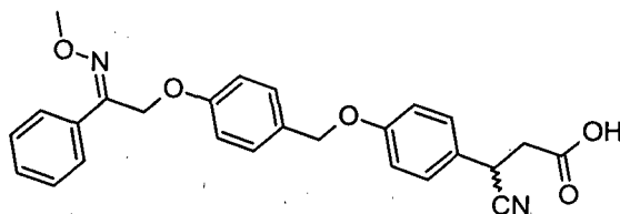
99 (Enantiomer-1)
