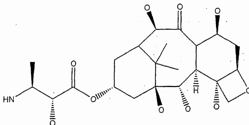
(VII).
