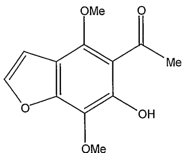
Khellinone
