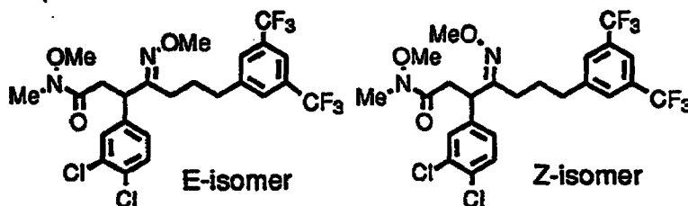
(9-3E, 9-3Z)
