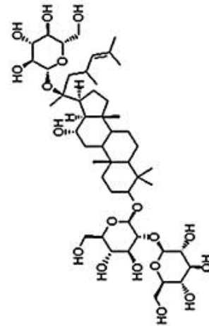
Ginsenoside Rd
