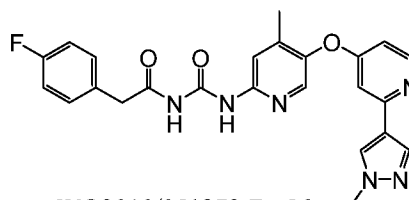
WO2010/051373 Ex 56
