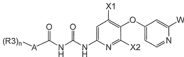
Formula Ic
