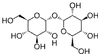
trehalose
