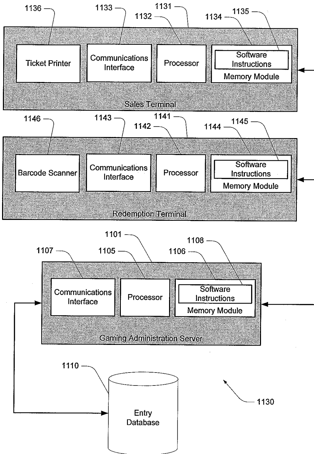
FIG. 11C
