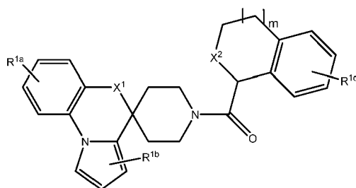
Formula VII-1
