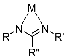
i) Amidinate ligand
