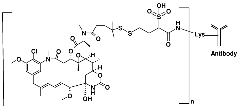
Ab-SulfoSPDB-DM4
