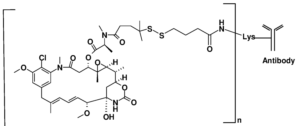
Ab-SPDB-DM4
