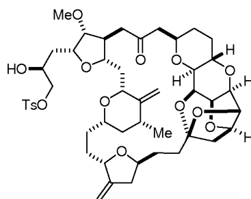
ER-082892
