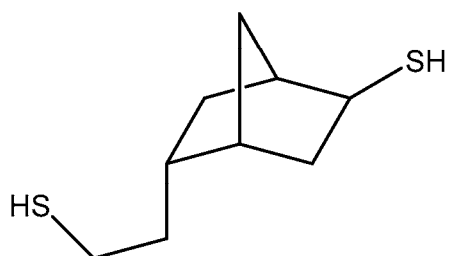
5-(2-mercaptoethyl)-norbornane-2-thiol
