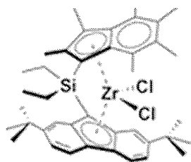
Et 2 SB(tBu 2 Flu, I*)ZrCl 2
