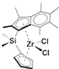
SB(Cp, I*)ZrCl 2
