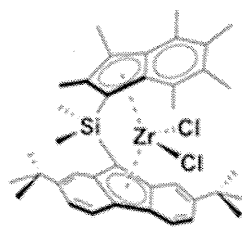
SB(tBu 2 Flu, I*)ZrCl 2
