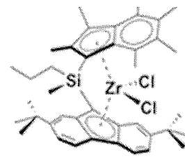
SB(tBu 2 Flu, I*)ZrCl 2
