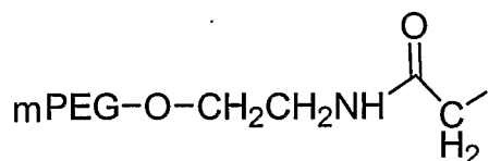
mPEG-iodoacetamide
