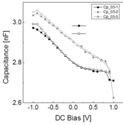
① : \text{ZrO}_x
