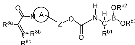
Formula I(d)
