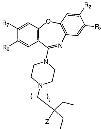
(IVc);
