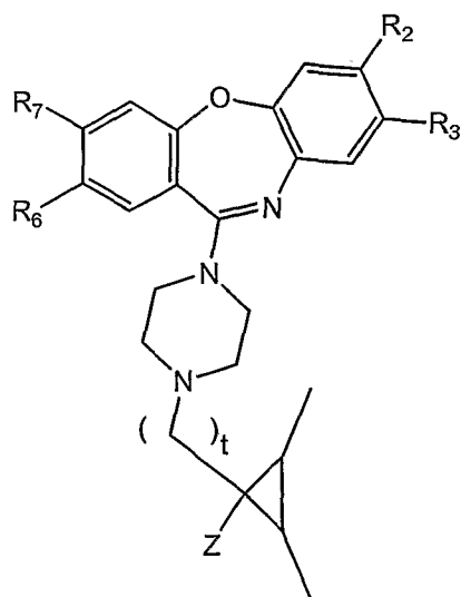
(IVd);
