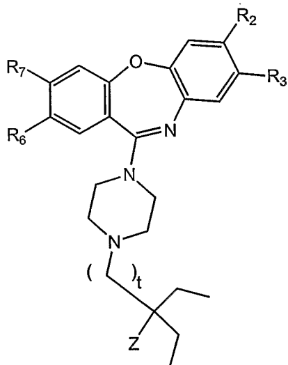
(IVc);
