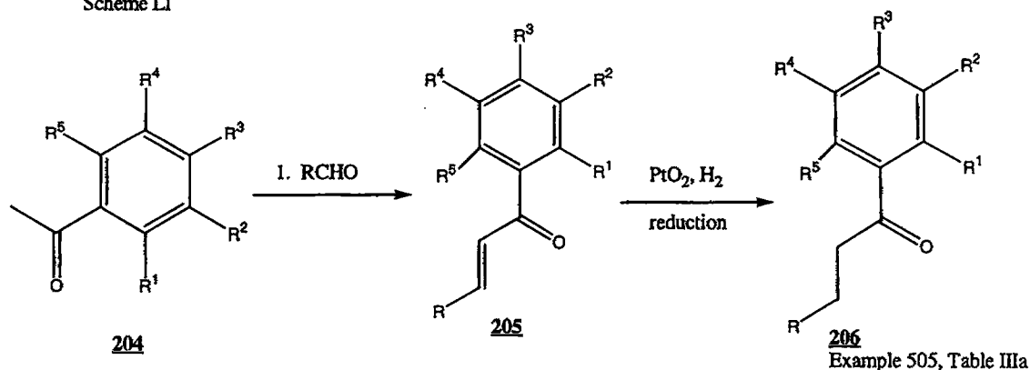
Scheme LI
