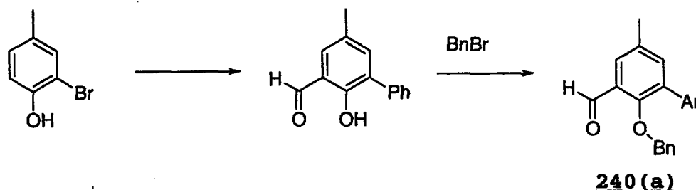
Scheme LX(1)
