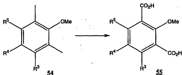
Scheme XIII :
