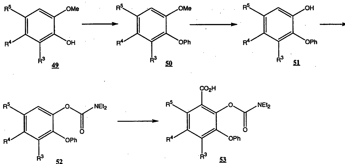
Scheme XII:
