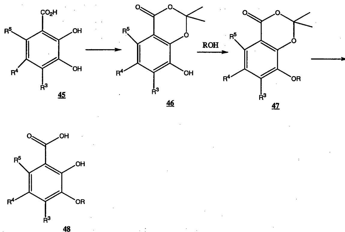
Scheme XI:
