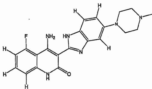
Tautomer IIIBb
