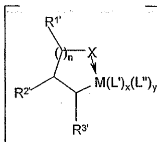
Structure Va
