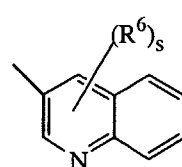
(a-24)
