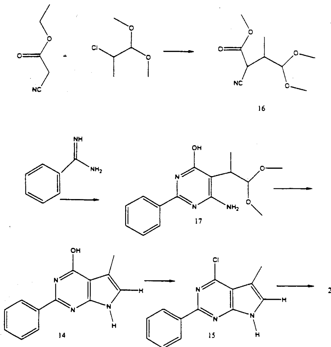
Scheme VI
