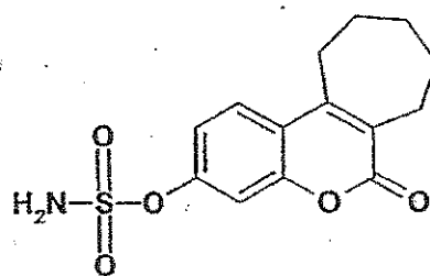
6,6,7 COUMATE
