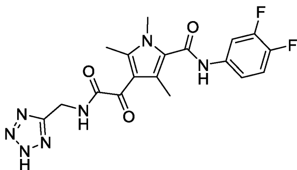
4-(2-(((2H-tetrazol-5-yl)methyl)amino)-2-oxoacetyl)-N-(3,4-difluorophenyl)-1,3,5-trimethyl-1H-pyrrole-2-carboxamide ( 82 )
