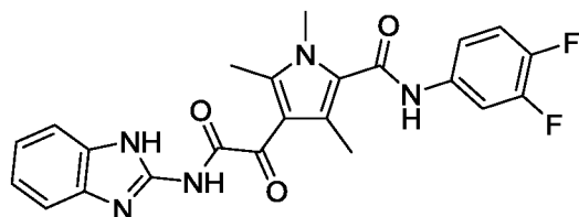
4-(2-((1H-benzo[d]imidazol-2-yl)amino)-2-oxoacetyl)-N-(3,4-difluorophenyl)-1,3,5-trimethyl-1H-pyrrole-2-carboxamide (46)
