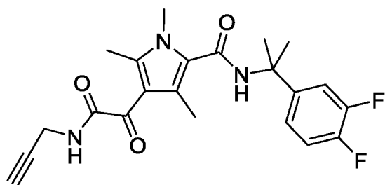
N-(2-(3,4-difluorophenyl)propan-2-yl)-1,3,5-trimethyl-4-(2-oxo-2-(prop-2-yn-1-ylamino)acetyl)-1H-pyrrole-2-carboxamide (56)
