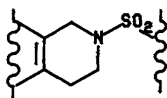
Sulfonamides
