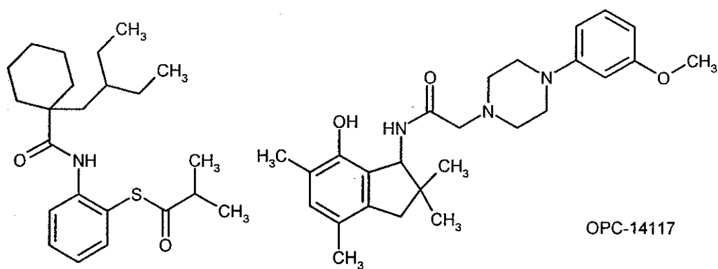
JTT-705
