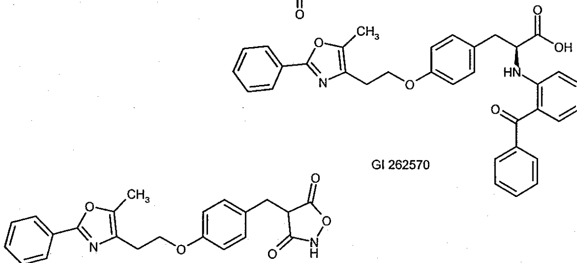
BMS-188494
