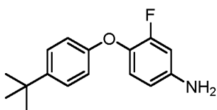
4-(4-(tert-butyl)phenoxy)-3-fluoroaniline,
