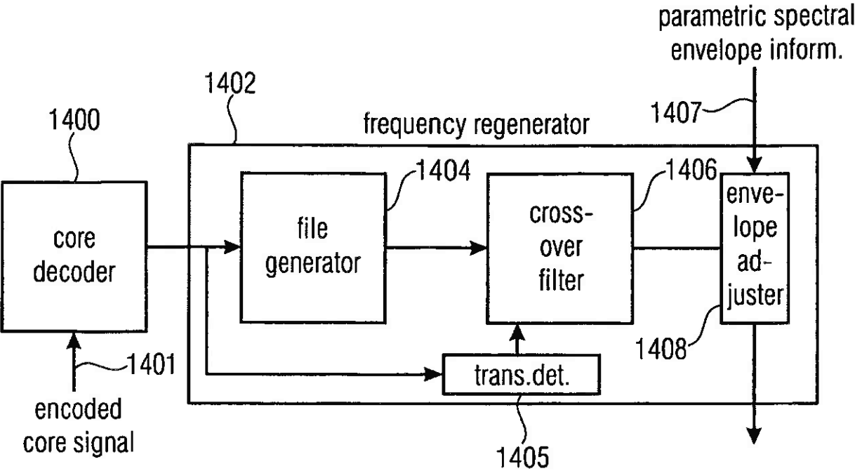
FIG 14A
