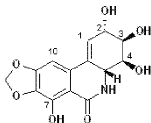
Narciclasine 1
