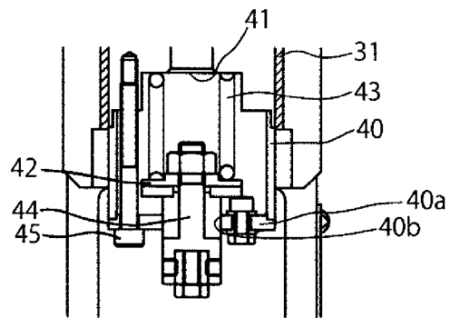
A詳細図
