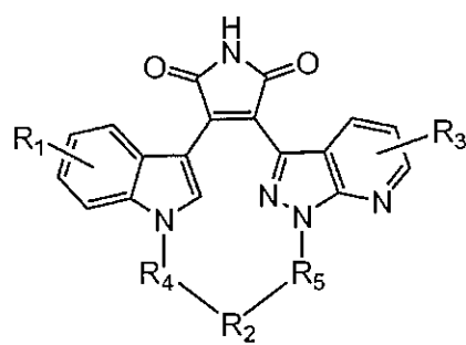
Formula (IIIk)
