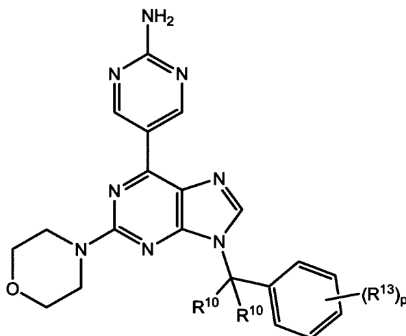
Formula (Va)
