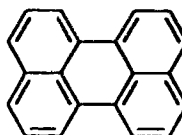
Perylene*
