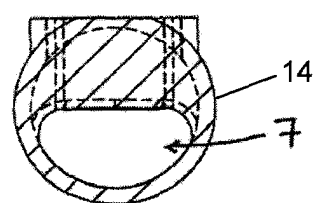
G-G (2 : 1)
