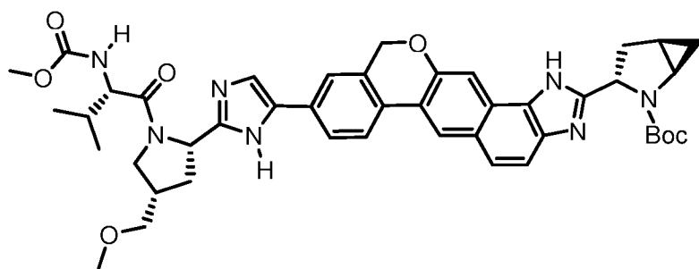
(1R,3S,5R)-tert-butyl 3-(9-(2-((S)-1-((S)-2-(methoxycarbonylamino)-3-methylbutanoyl)-4-methoxymethylpyrrolidin-2-yl)-1H-imidazol-5-yl)-1,11-dihydroisochromeno[4',3':6,7]naphtho[1,2-d]imidazol-2-yl)-2-azabicyclo[3.1.0]hexane-2-carboxylate
