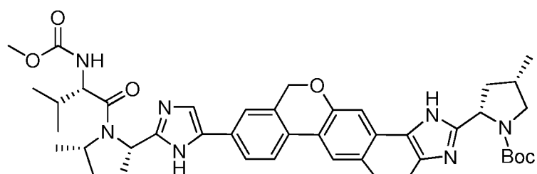
tert-butyl (2S,4S)-2-[9-(2-((2S,4S)-1-[N-(methoxycarbonyl)-L-valyl]-5-methylpyrrolidin-2-yl)-1H-imidazol-5-yl)-1,11-dihydroisochromeno[4',3':6,7]naphtho[1,2-d]imidazol-2-yl]-4-methylpyrrolidine-1-carboxylate
