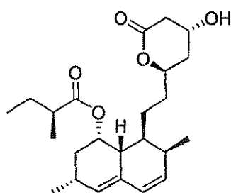
Lovastatin lactone
