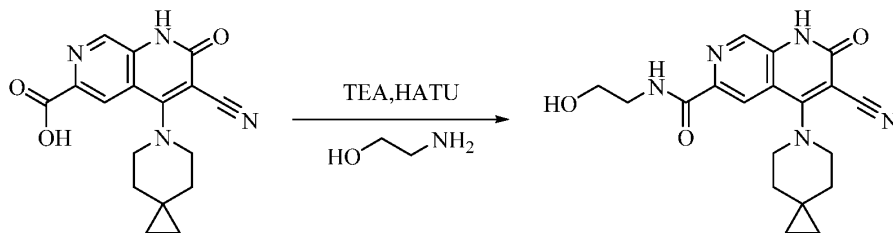
化合物 97
