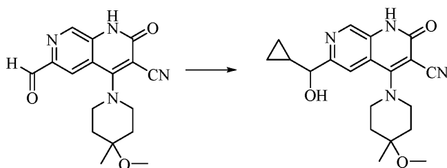
化合物 130
