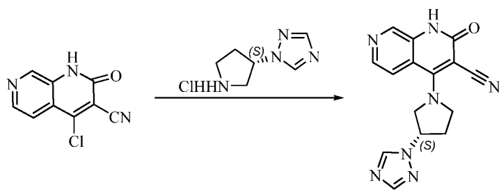
化合物 112
