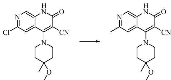
化合物 158
