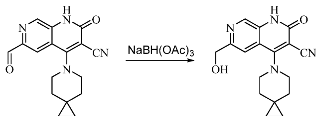
化合物 62
