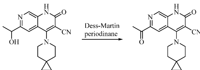
化合物 95
