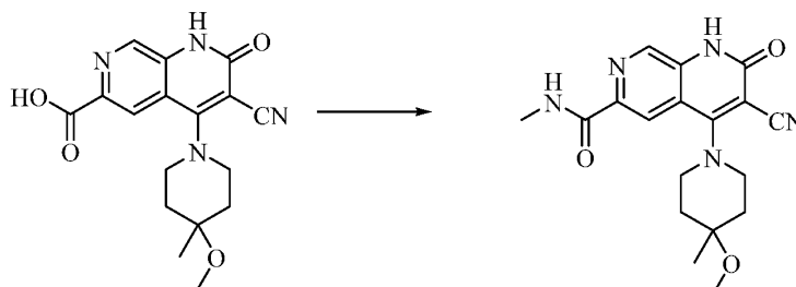
化合物 131
