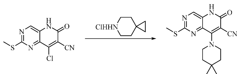
化合物 129
