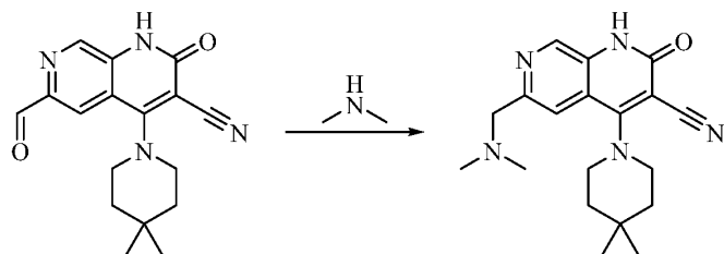
化合物 48
