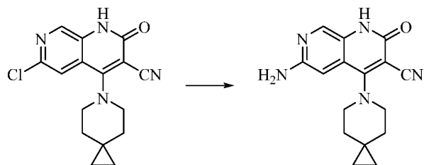
化合物 44
