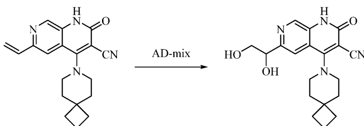
化合物 33
