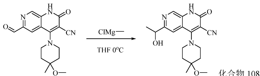
化合物 108
