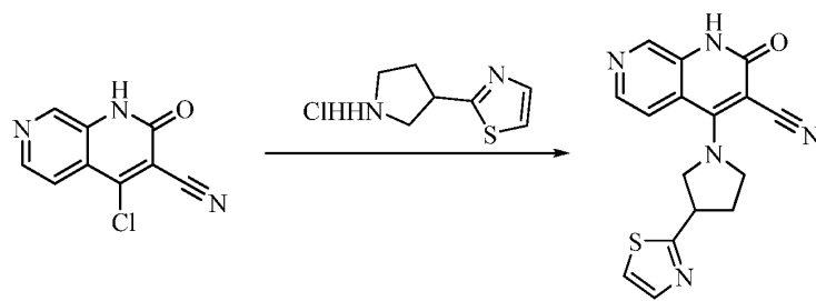
化合物 113
