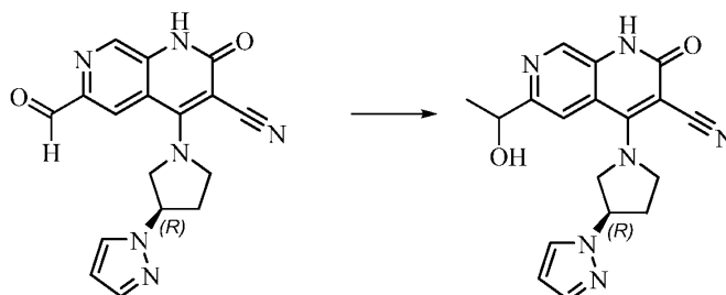
化合物 156
