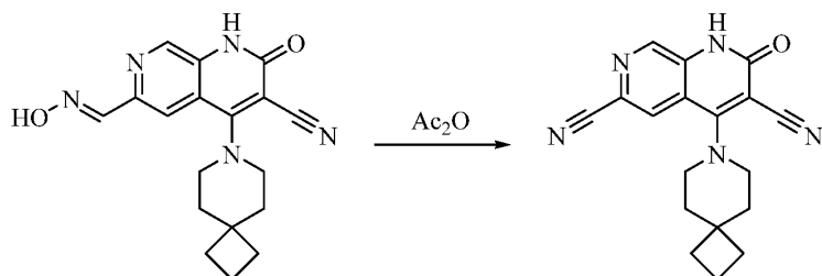
化合物 77
