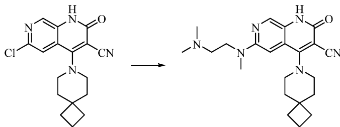
化合物 61
