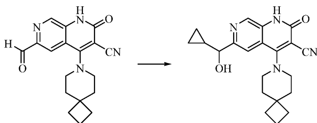
化合物 160
