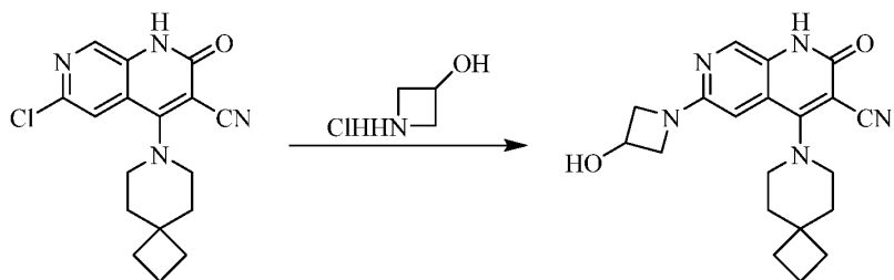
化合物 51
