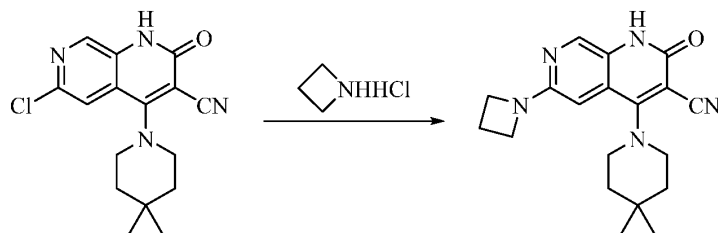
化合物 49
