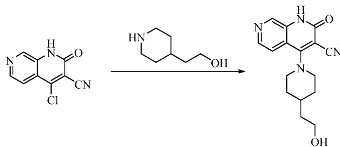
化合物 28
