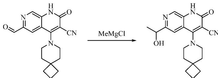
化合物 94
