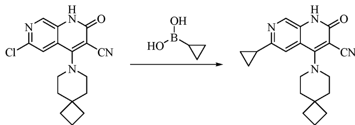
化合物 60
