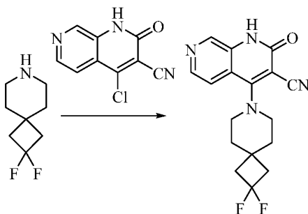
化合物 43
