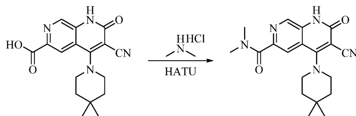
化合物 149
