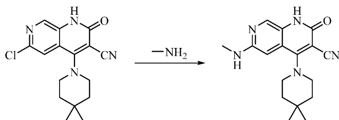
化合物 45
