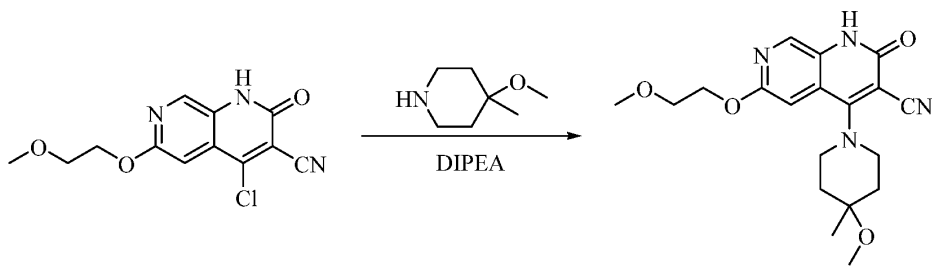
化合物 145
