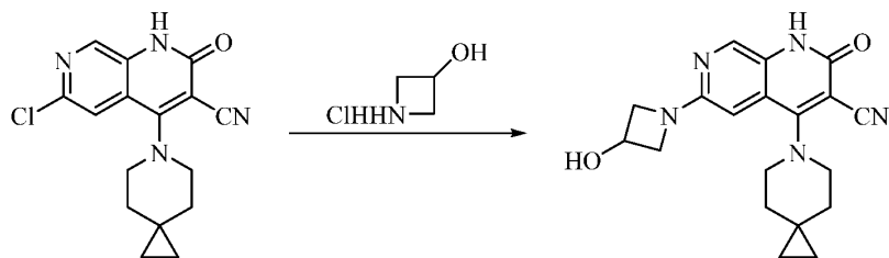
化合物 50
