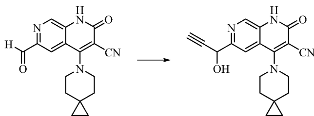
化合物 91
