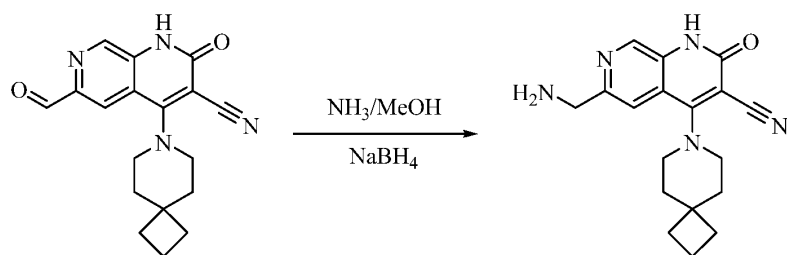
化合物 78
