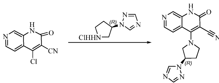
化合物 154
