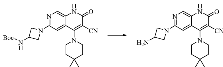
化合物 52
