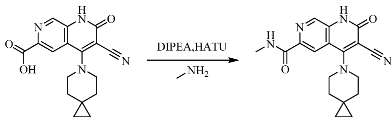
化合物 96
