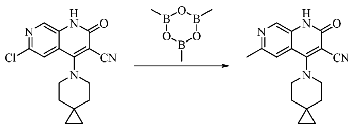
化合物 63
