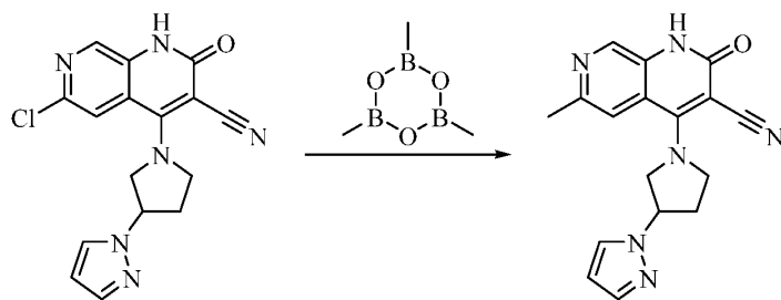
化合物 27
