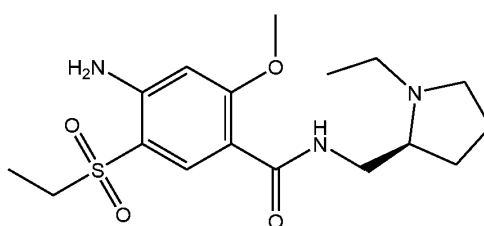
S-4-Amino-N-[(1-ethyl-2-pyrrolidinyl)methyl]-5-(ethylsulfonyl)-2-methoxybenzamide
