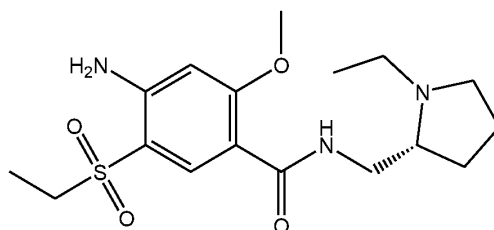
R-4-Amino-N-[(1-ethyl-2-pyrrolidinyl)methyl]-5-(ethylsulfonyl)-2-methoxybenzamide,
