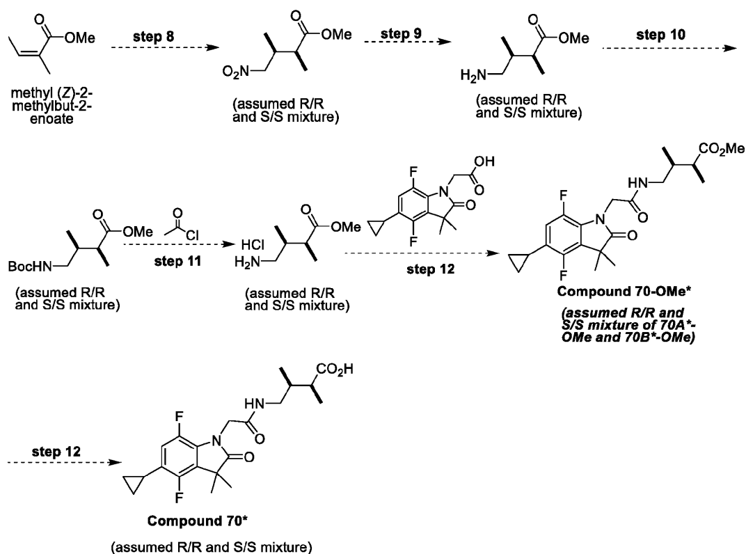
Scheme 25B.
