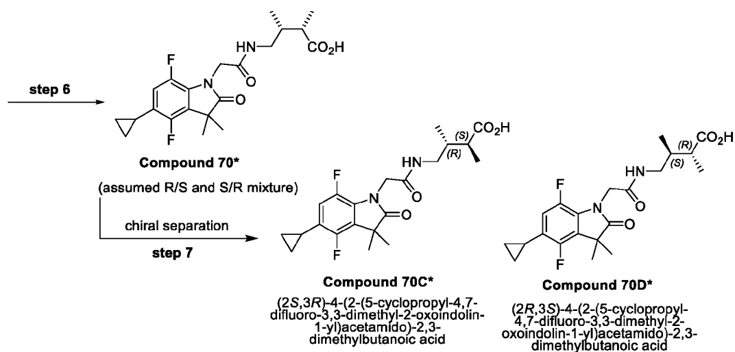
Scheme 25B.
