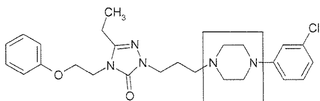
Nefazodone
