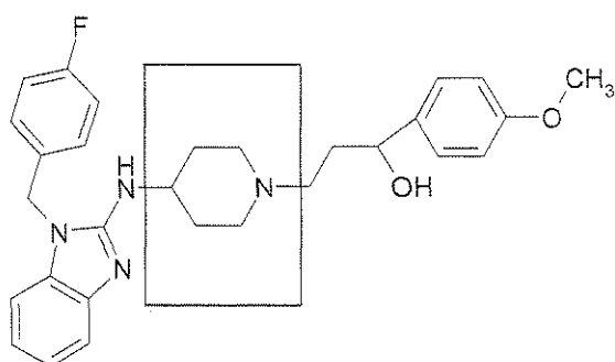
Astemizole
