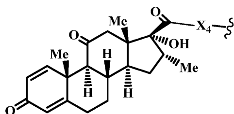
LB33 (Prednisone),
