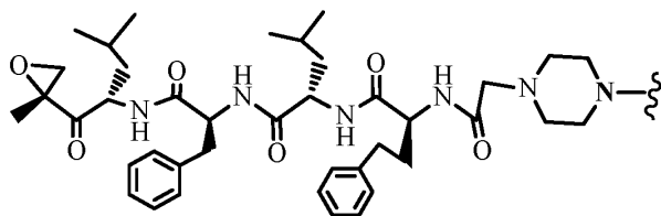
LB40 (Carfilzomib analog),
