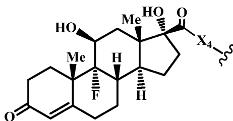
LB28 (Fludrocortisone),
