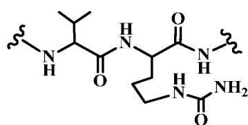
valine-citrulline (val-cit),
