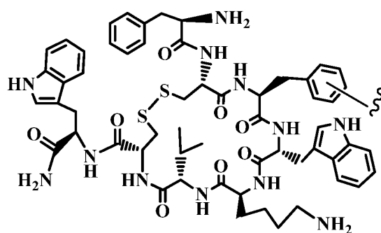
LB09 (Vapreotide (Sanvar), a Somatostatin ana-
