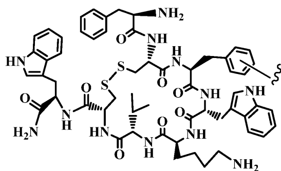
LB09 (Vapreotide (Sanvar), a Somatostatin
