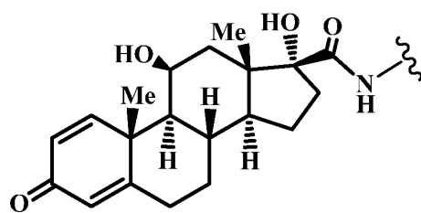
LB34 (Prednisolone),
