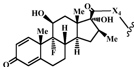
LB36 (Betamethasone),
