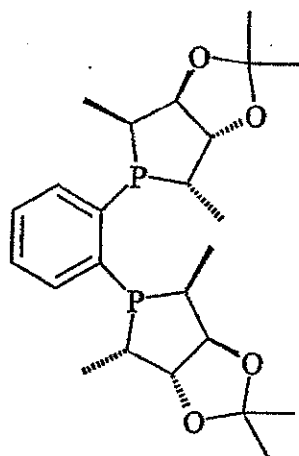
( S,S,S,S )-"Me-KetalPhos",
