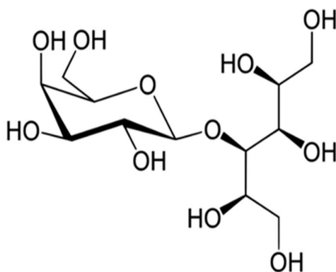
Lactitol;
