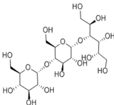
Maltotritol;
