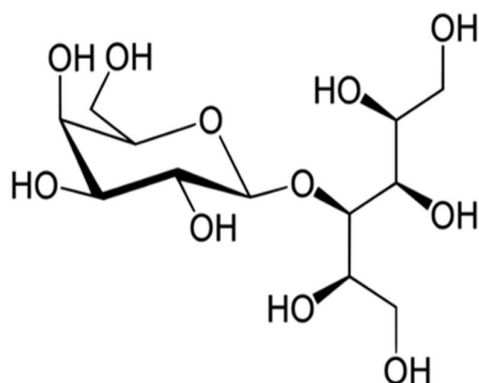
Lactitol;
