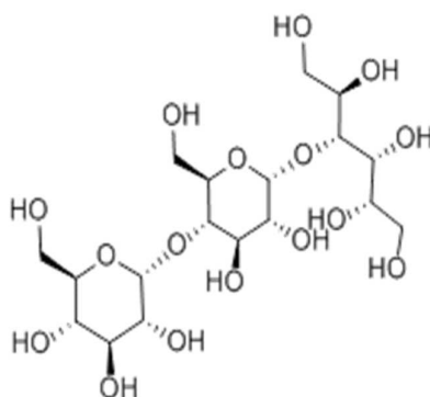
Maltotritol;
