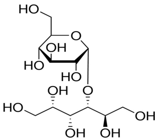
Maltitol; or
