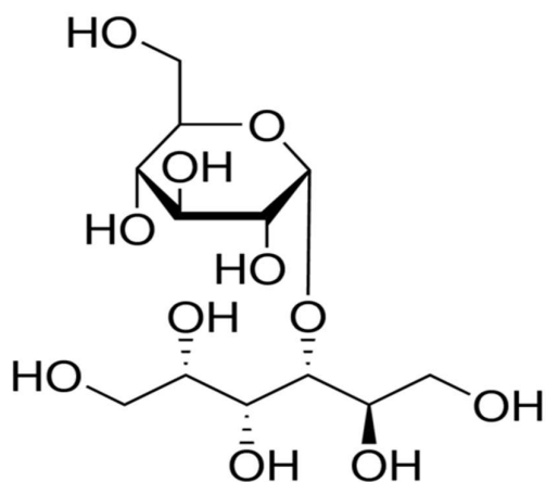
Maltitol; or
