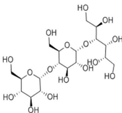
Maltotrititol;
