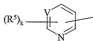
XXXXI
