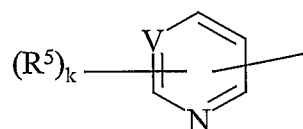
XXXXI
