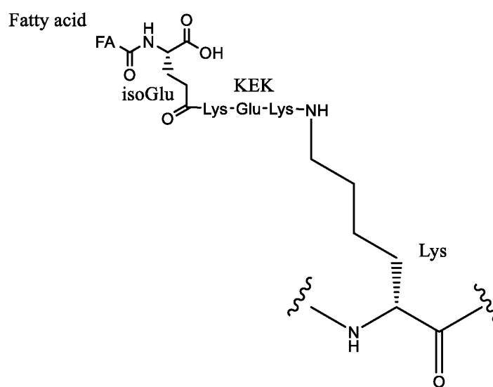
[K([Fatty acid]-isoGlu-KEK)]
