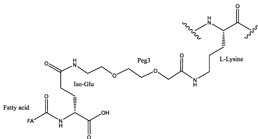
[K([Fatty acid]-isoGlu-Peg3)]
