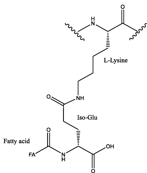
[K([Fatty acid]-isoGlu)]
