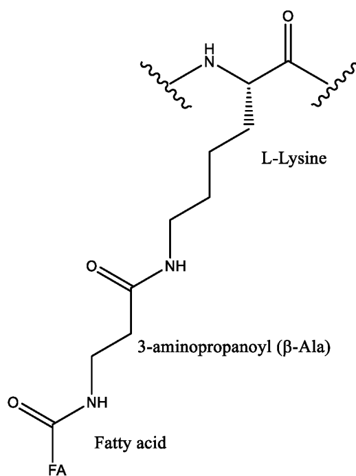
[K([Fatty acid]-isoGlu)]
