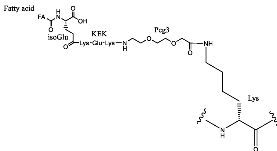
[K([Fatty acid]-isoGlu-KEK-Peg3)]
