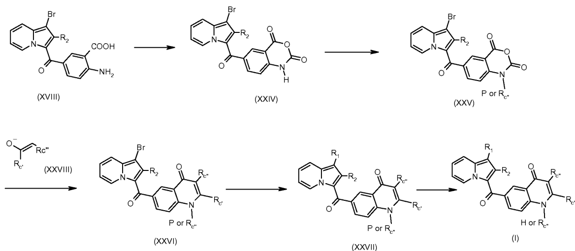
Scheme 6 (Method 6):
