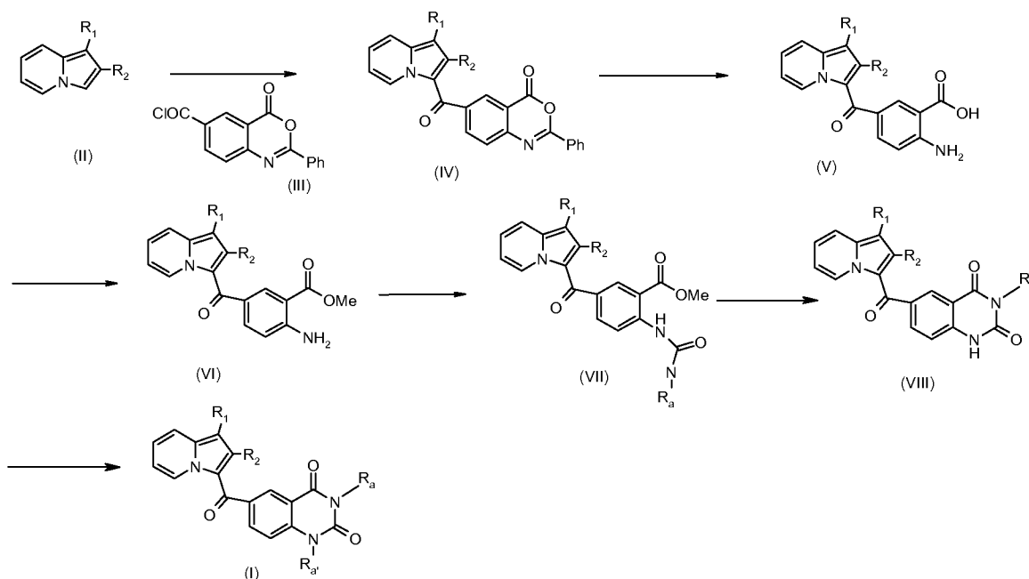
Scheme 1 (Method 1):
