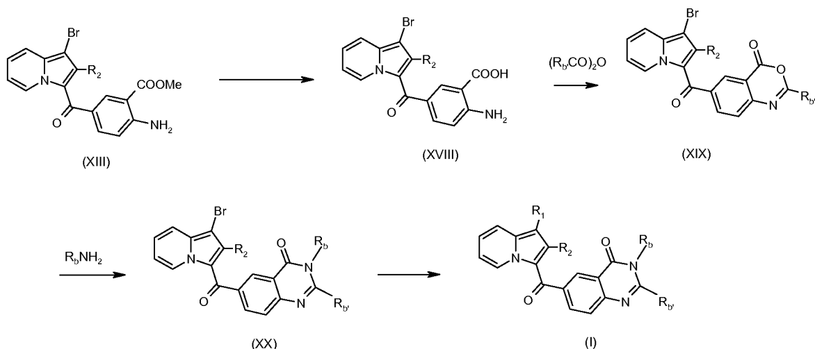
Scheme 4 (Method 4):
