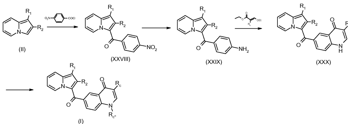
Scheme 7 (Method 7):
