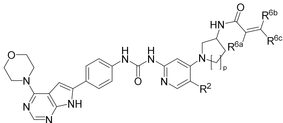
(VIa);
