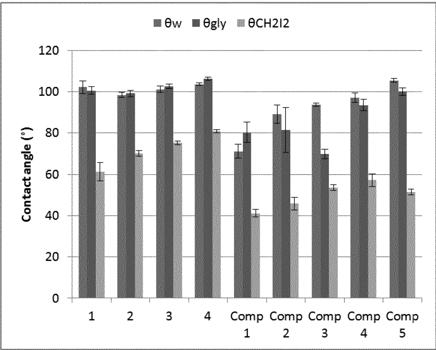
Figure 2 : Contact angles values
