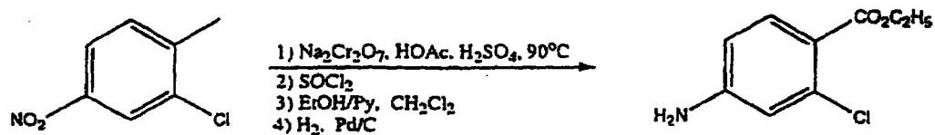
Compound E1
