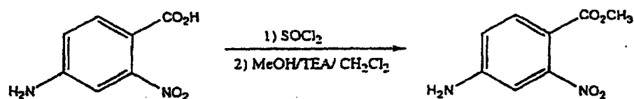
Compound F1
